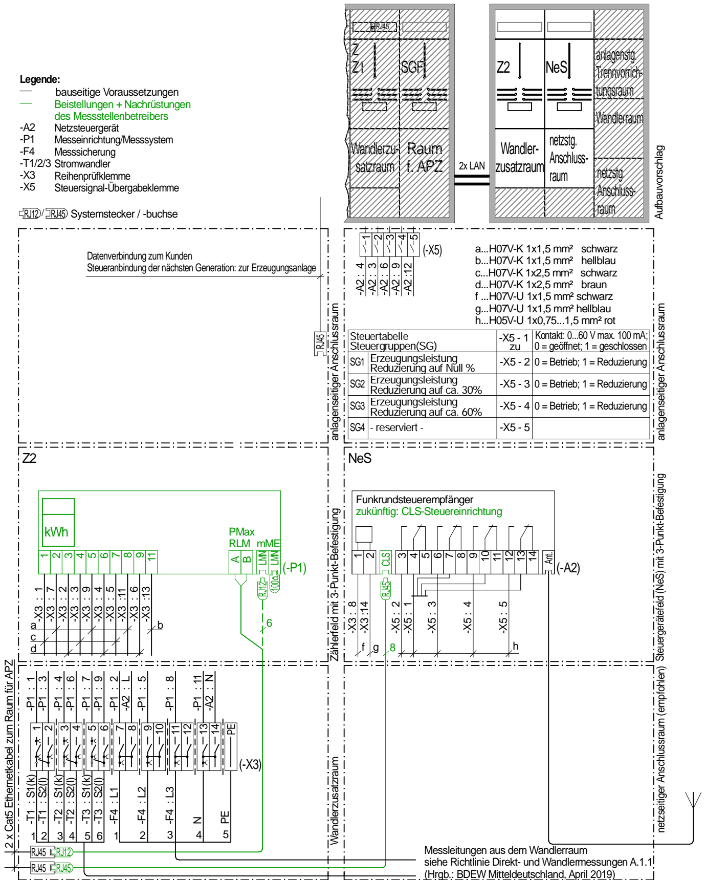
Bild 2 Aufbau Zählerplatz / NeS-Platz (Wandlermessung)
