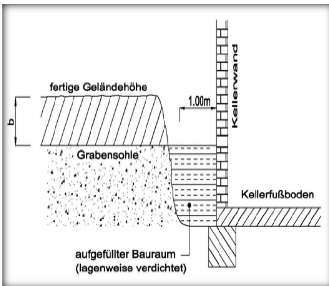
Bild2: Verdichtung im Bereich Keller, Bodenplattenverfüllung
