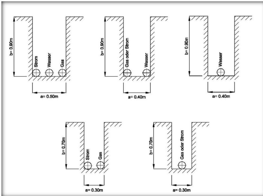
Bild 3: Mustergräben
