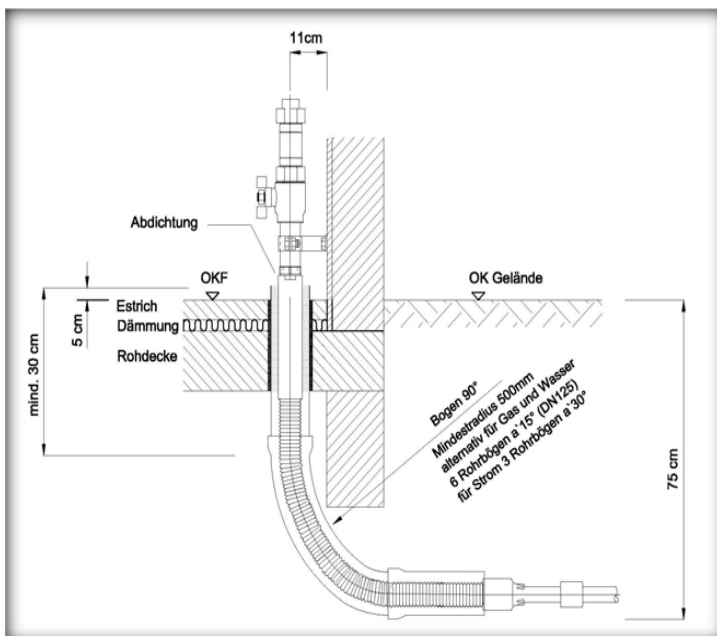
Bild 5: Gashauseinführung in ein nicht unterkellertes Gebäude
